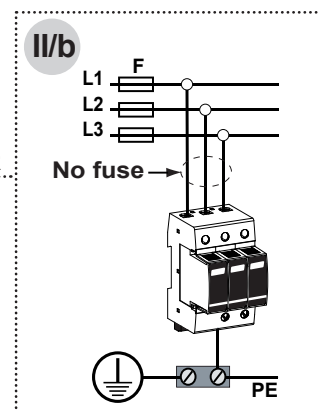
CITEL DACF15S-30-440
